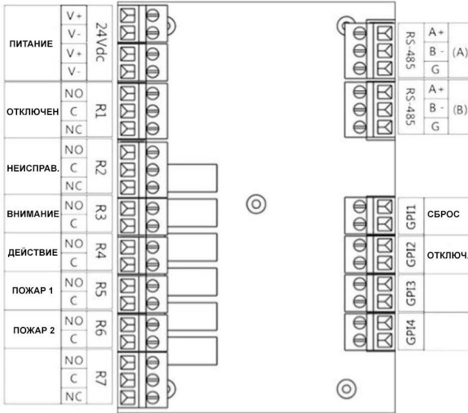
Рисунок 4.5 – Расположение терминалов на коммуникационной плате
