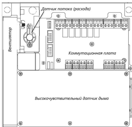
Рисунок 4.2 – Конструкция извещателя
