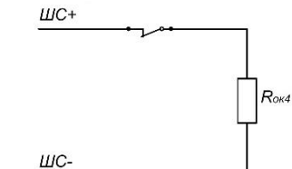
Рисунок 4.7 – Схема подключения реле «Неисправность»
