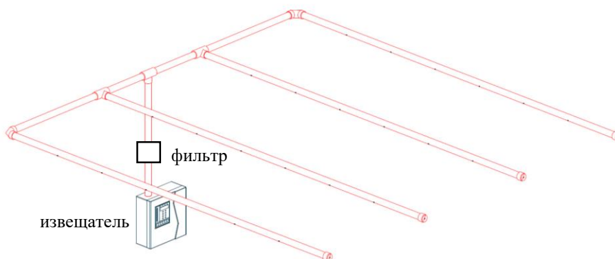
Рисунок 4.3 – Структура воздухопровода с четырьмя трубами
