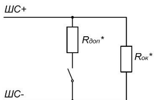
Рисунок 4.6 – Схема подключения реле «Внимание», «Действие», «Пожар 1», «Пожар 2»
