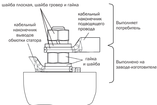
Рисунок 5 – Схема контактного соединения
