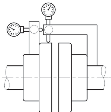
Рисунок 8 – Схема комбинированного измерения аксиальной и радиальной несоосности
