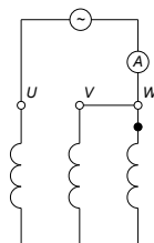
Рисунок 4 – Схема соединения обмоток «Y» при сушке
