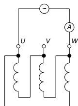
Рисунок 3 – Схема соединения обмоток «Δ» при сушке
