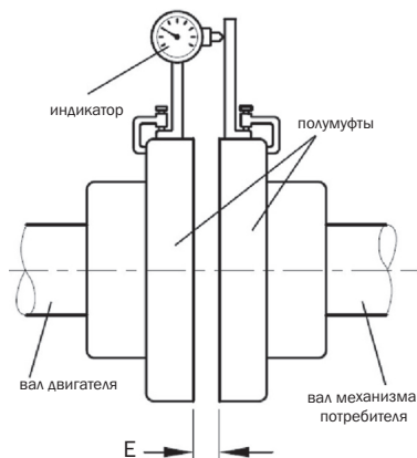
Рисунок 6 – Схема измерения аксиальной несоосности
