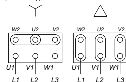
Схема соединений на панели
