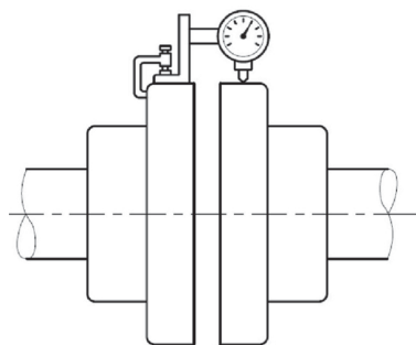
Рисунок 7 – Схема измерения радиальной несоосности (смещения осей)
