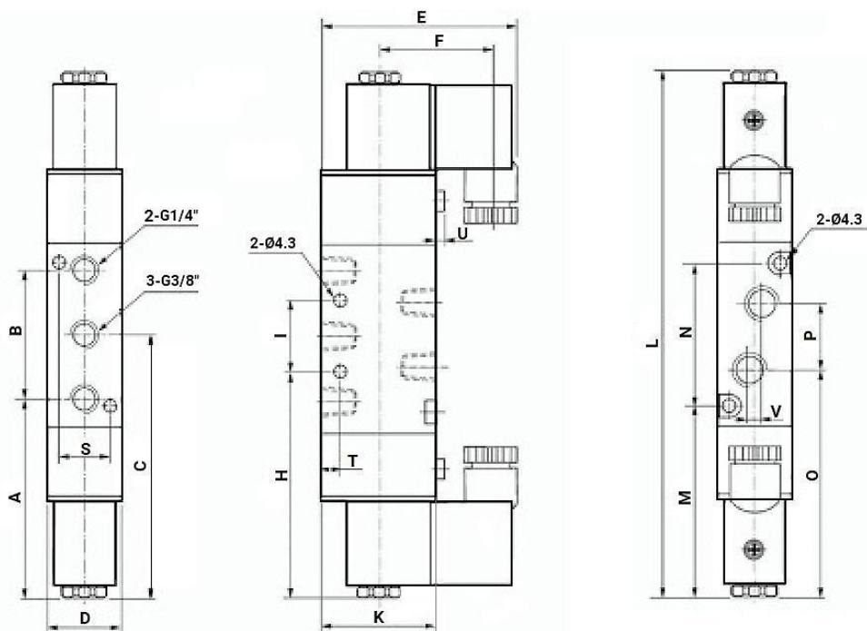
Рисунок 3 – Размеры PND1-S2EM-52-2-T10-220VAC
