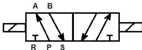
Рисунок 4 – Схема работы
