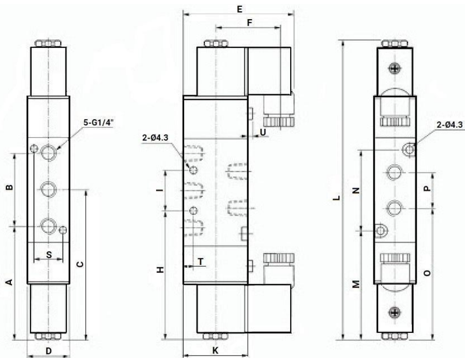
Рисунок 2 – Размеры PND1-S2EM-52-2-T08-220VAC
