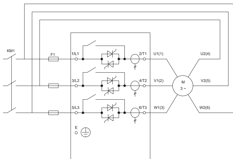
КМ1 – главный контактор F1 – полупроводниковый предохранитель
