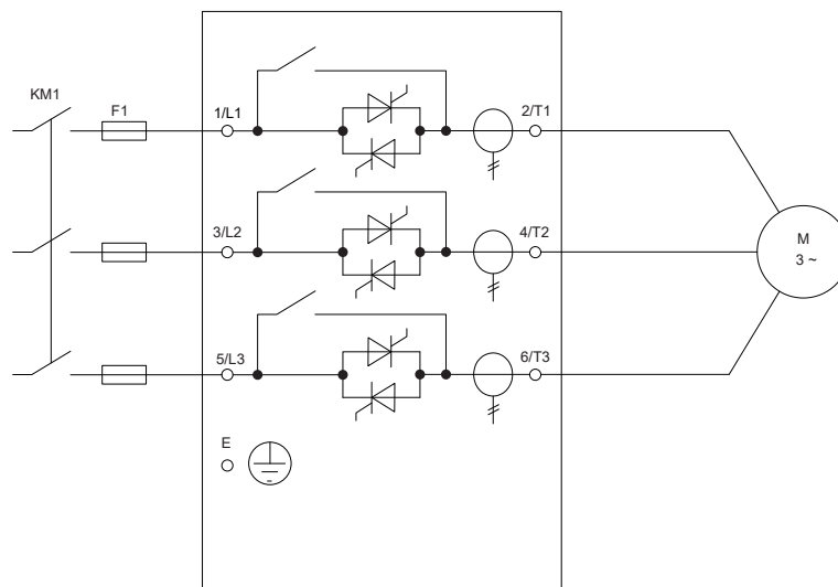
КМ1 – главный контактор F1 – полупроводниковый предохранитель
