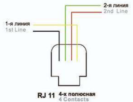
Схема цепи / Wiring Diagram
