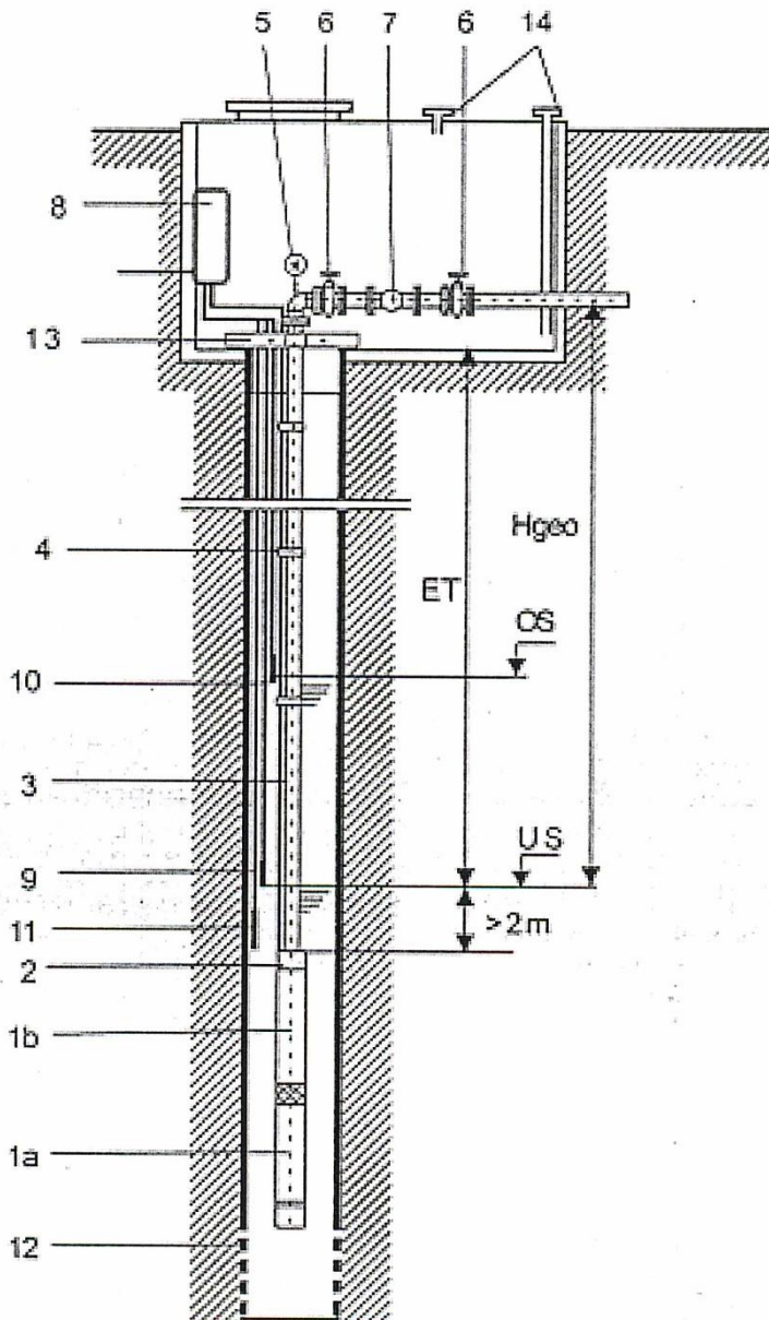
Рисунок 12. Пример установки агрегата электронасосного в скважину
