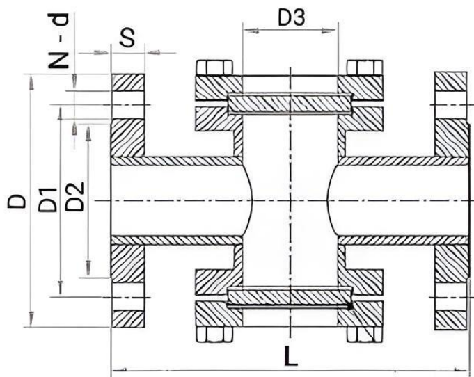
Рисунок 2 - Размеры
