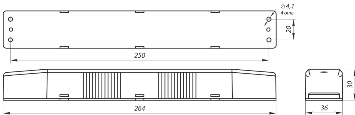
Рис.7 Габаритные и присоединительные размеры источника аварийного питания STABILAR3.LED
