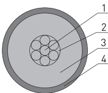
Рисунок 1 – Конструкция токоотвода
