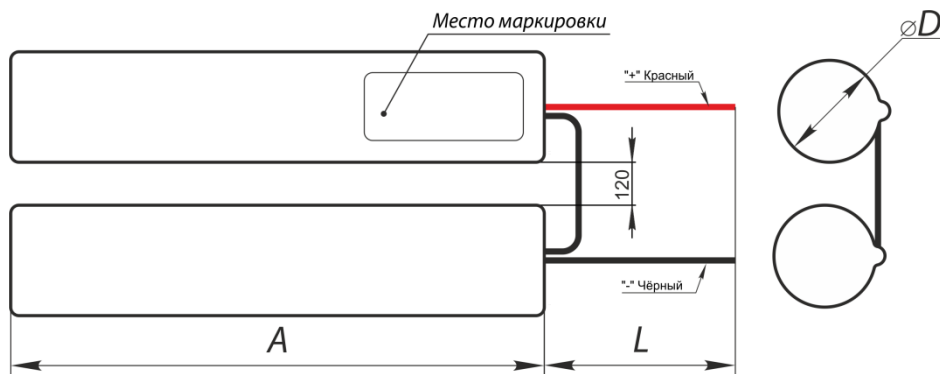
Рис.8 Габаритные размеры батареи
