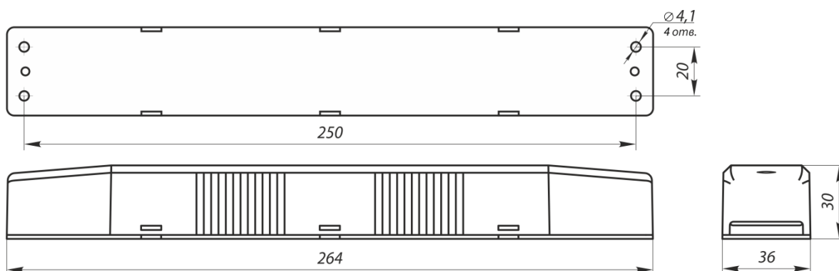
Рис. 7 Габаритные и присоединительные размеры источника аварийного питания STABILAR3.LED
