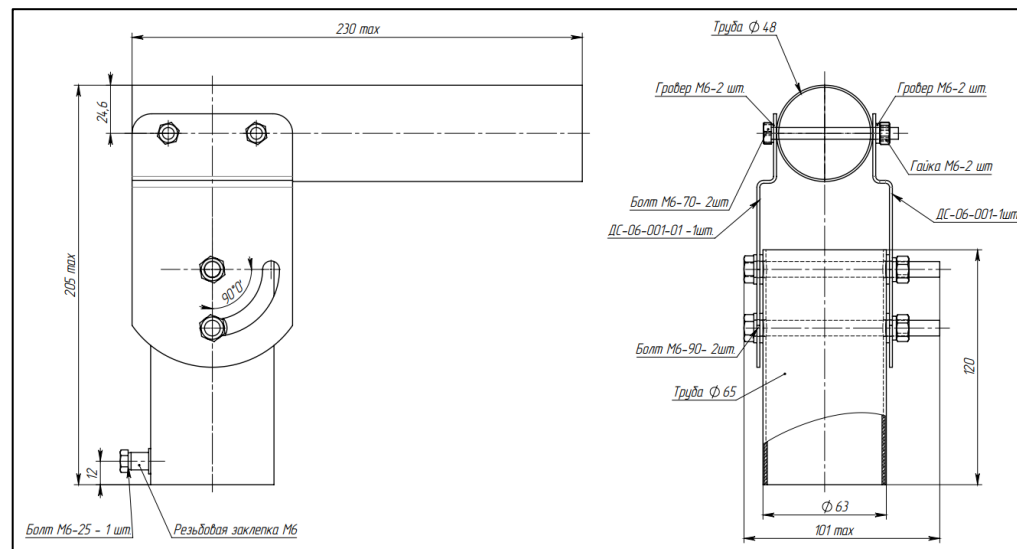
Рисунок 1. Сборочный чертёж ДС-06-48
