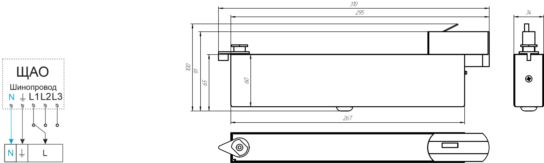
Рис. №1 Схема подключения к групповой цепи питания.
