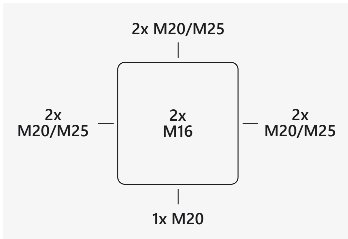
Схема расположения выбивных отверстий
