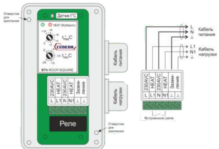
Схема подключения
