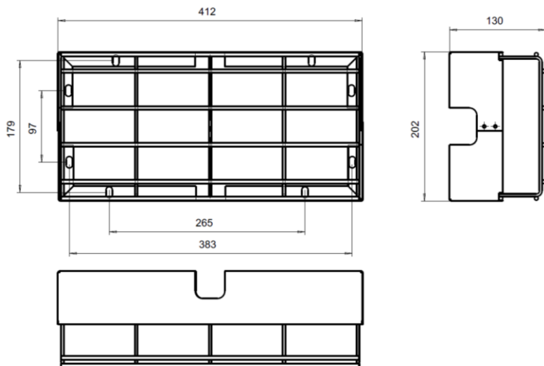
Рис. №3 Аксессуары. Решётка защитная BS-R-1 (а2333)
