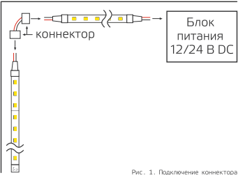
Рис. 1. Подключение коннектора
