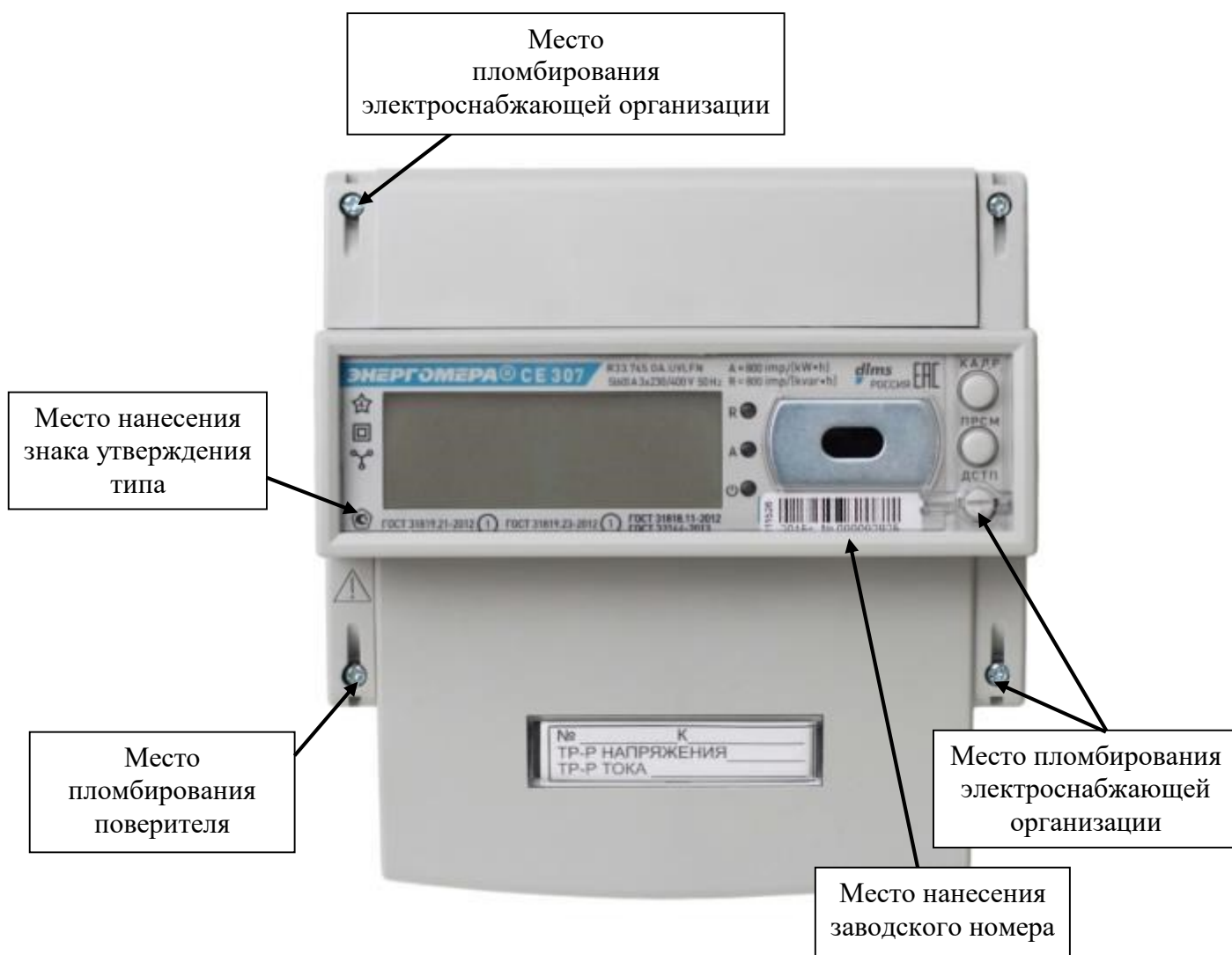
Рисунок 3 – Общий вид счетчика SE307 R33*
