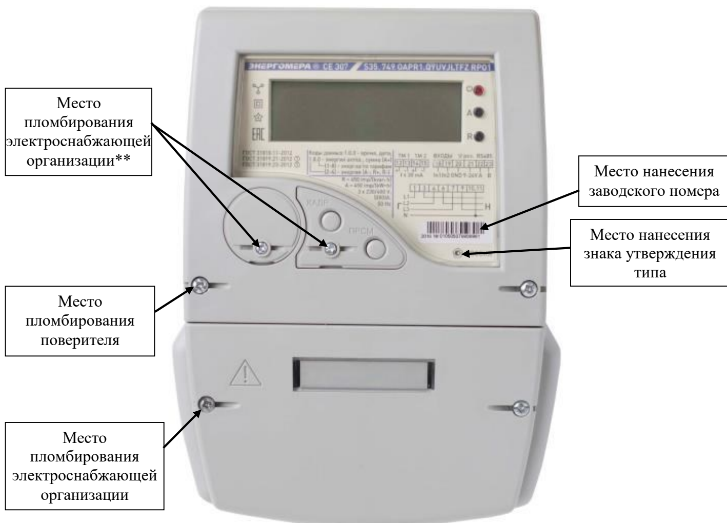
Рисунок 6 – Общий вид счетчика СЕ307 S35 исполнение 1*
