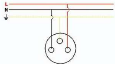
Схема цепи / Wiring Diagram
