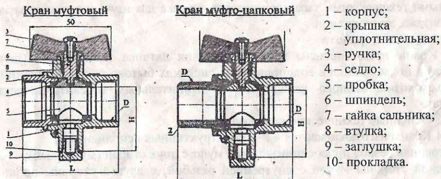
Рисунок 1. Краны шаровые для подключения датчика температуры.
