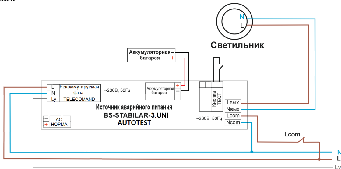
Рис. 1б Схема подключения BS-STABILAR3-81-B1-UNI AUTOTEST для аварийного светового прибора с люминесцентными лампами с электронными ПРА в универсальном режиме:
