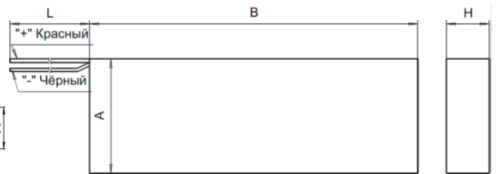
Рис.8 Батарея BS-10HRHT14/50-1.6/F-HB500-VHR-3N-1
