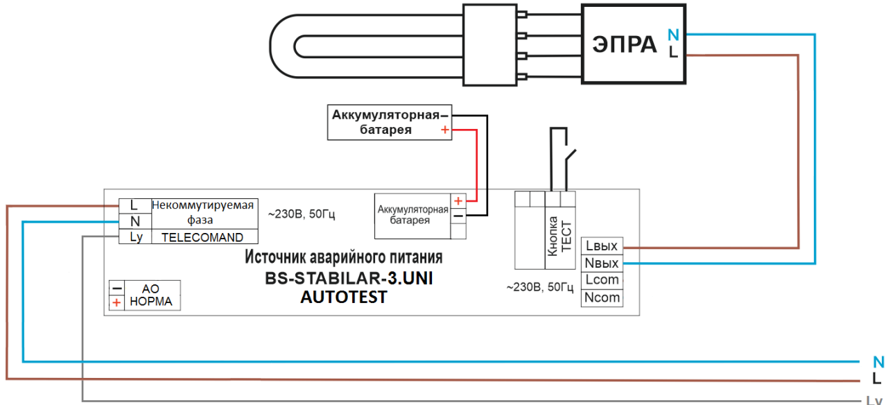
СХЕМЫ ПОДКЛЮЧЕНИЯ К ГРУППОВЫМ ЦЕПЯМ ПИТАНИЯ И УПРАВЛЕНИЯ СВЕТОВЫХ ПРИБОРОВ ОБОРУДОВАННЫХ БАП.
