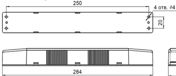
Рис. 7 Блок аварийного питания BS-STABILAR3-81-B1-UNI AUTOTEST
