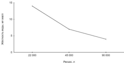
Рис.1 График зависимости ресурса картриджа Thermex ION от жесткости воды
