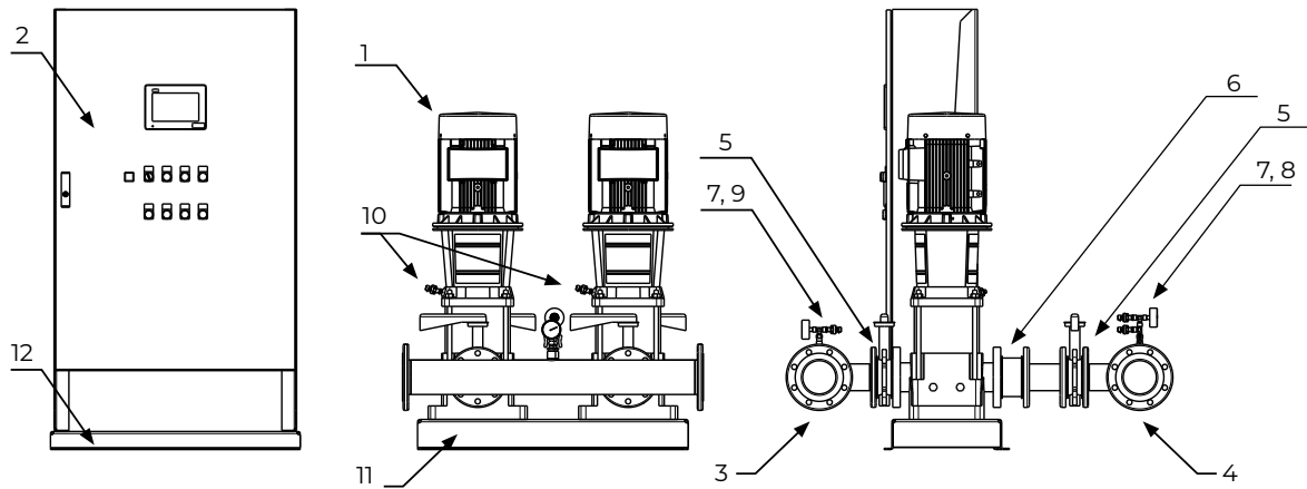
Рис. 4 Внешний вид станции пожаротушения HC-FS-V на примере системы с одним основным и одним резервным насосами ВМ
