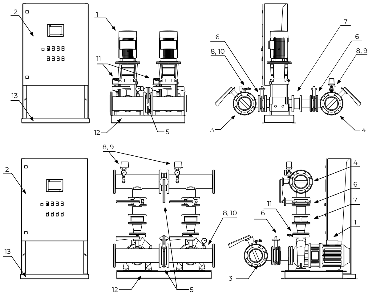
Рис. 3 Пример внешнего вида станции пожаротушения HC-FS-A на примере системы с одним основным и одним резервным насосами ВМ и КМ(С)
