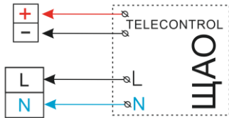
Рис. №1 Схемы подключения к групповой цепи питания и подключения к групповой цепи управления.
