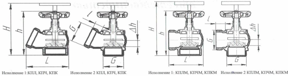
Рисунок 1—Внешний вид клапанов угловых моделей KPPL, KPCH, KPK и KPPLM, KPCHM, KPKM
