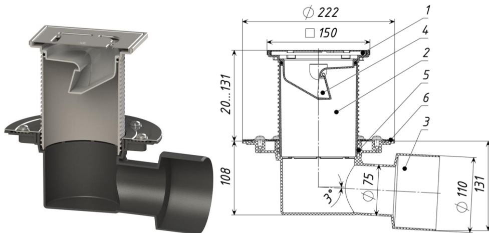
Рис. 1 ТП-5100.1N-3000 Трап с незамерзающим запахозапирающим устройством
