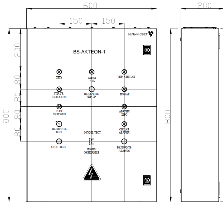
Рис. №2 Установочный чертёж.
