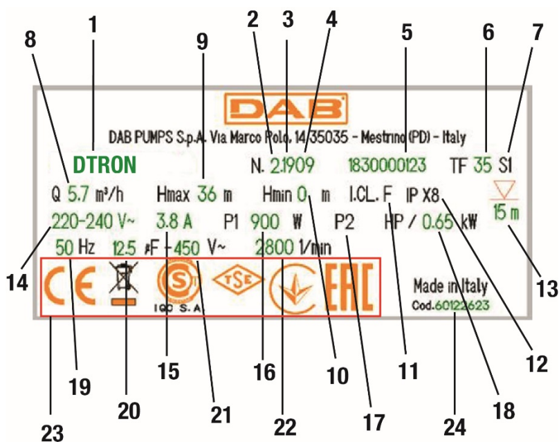
Εικ.4 Πινακίδα
