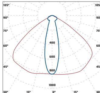
«Diora Quadro Store» специальная КСС 110°x30°
