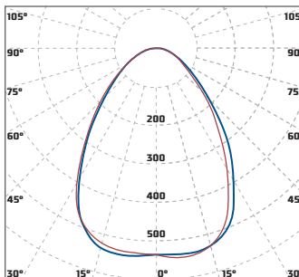
«Diora Quadro Г80» глубокая КСС 80°
