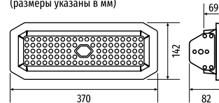
ДСП-112-00 97 Вт (размеры указаны в мм)
