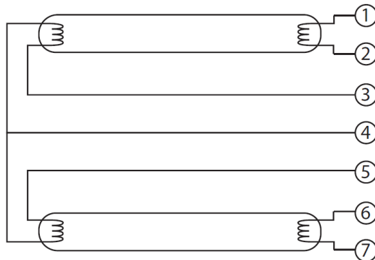
Рис. 2 Схема подключения ЭПРА EB52
