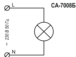
Рисунок 6. Схема подключения светильника CA-7008Б
