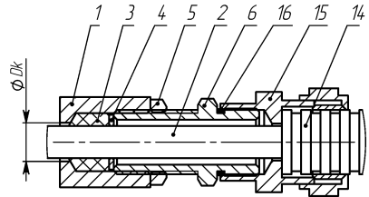
г) монтаж кабелем в металлорукаве в кабельном вводе KBM
