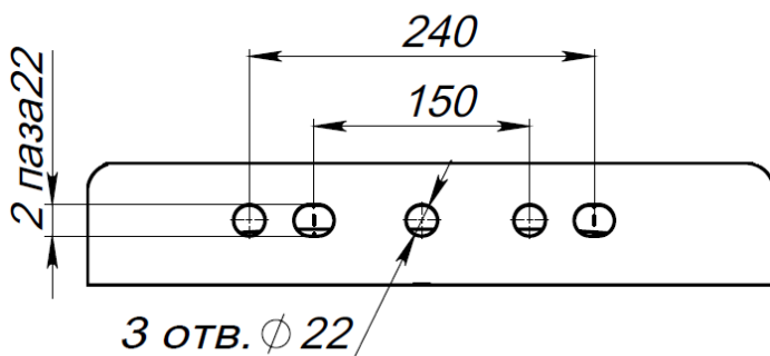
Монтажные отверстия
