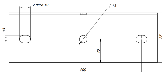
Монтажные отверстия
