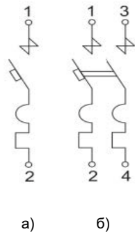
рис. 3. Принципиальные электрические схемы выключателей а) однополюсного; б) двухполюсного с двумя защищенными полюсами;
