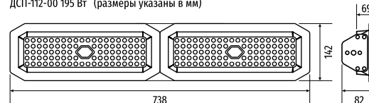
ДСП-112-00 195 Вт (размеры указаны в мм)
