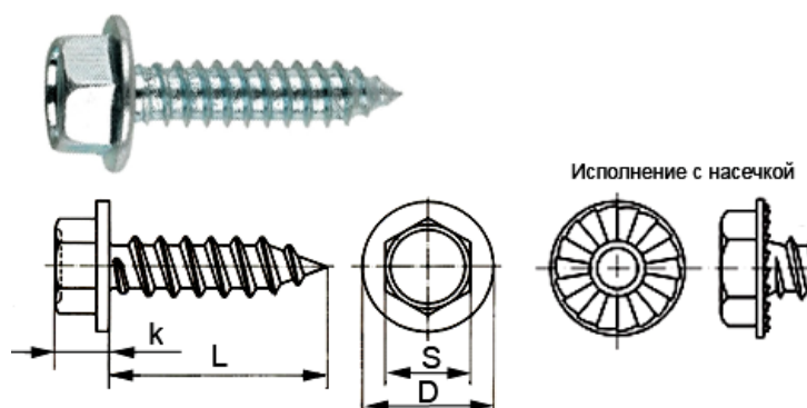
Размеры и характеристики DIN 6928 (EN ISO 7053)
