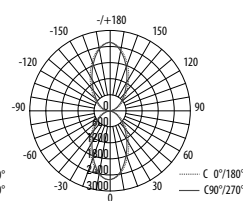
PWL-245110/24D 2x9W IP65
