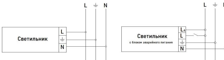
Рис. 2. Схемы подключения к сети
