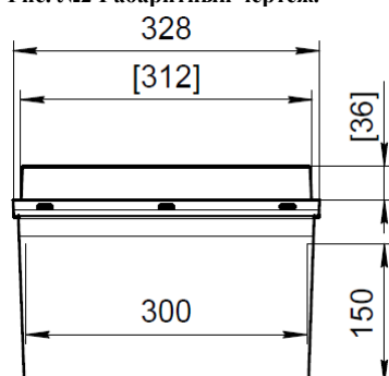
Рис. №2 Габаритный чертёж.
