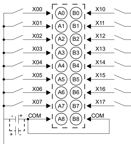
б) модуль IOD-430-TB-16NP000
