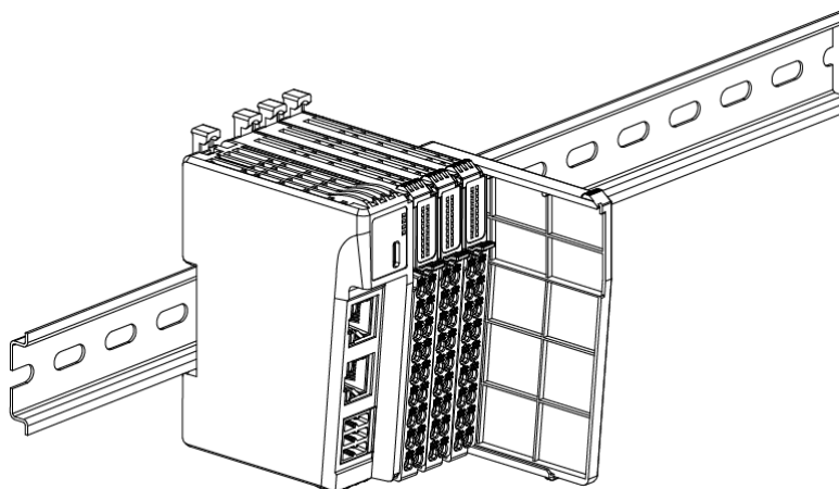
Рисунок 8 – Установка модуля клеммной крышки
