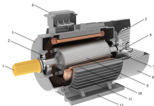
Рисунок 1 – Устройство двигателя:
