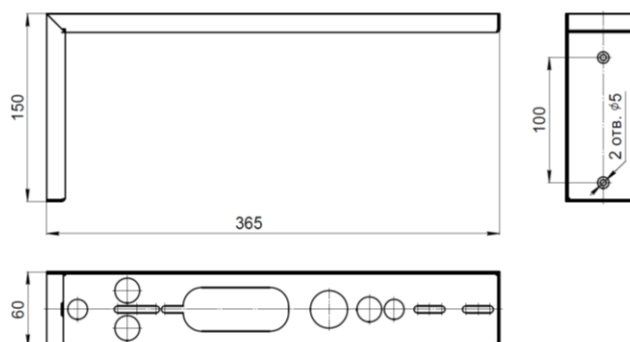
Рис. №6 Кронштейн BS-K-3
