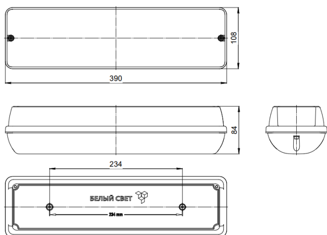
Рис. №5 Габаритный чертёж.
