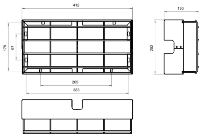
Рис. №7 Решётка защитная BS-R-1 (a2333)
