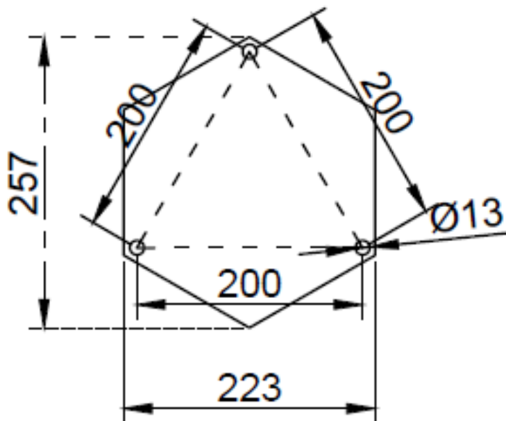
Схема основания светильника PL767
