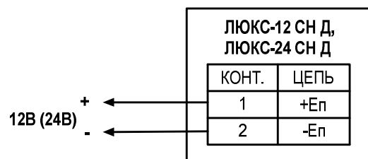
Рис.1. Схема подключения.
