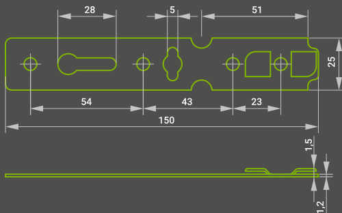
Анкерная пластина КВЕ
