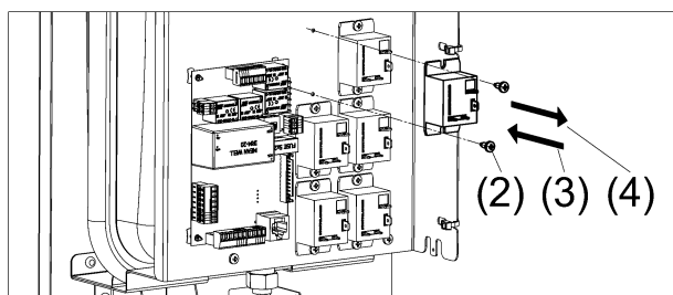
Рисунок 17. Замена реле
