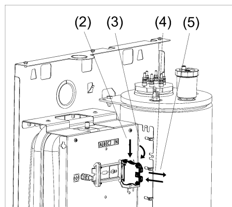
Рисунок 19. Замена клеммных колодок
