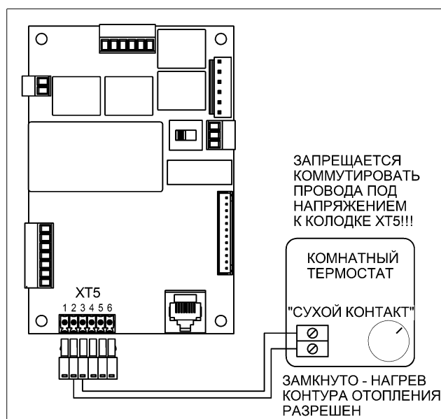
Рисунок 34. Схема подключения комнатного термостата
