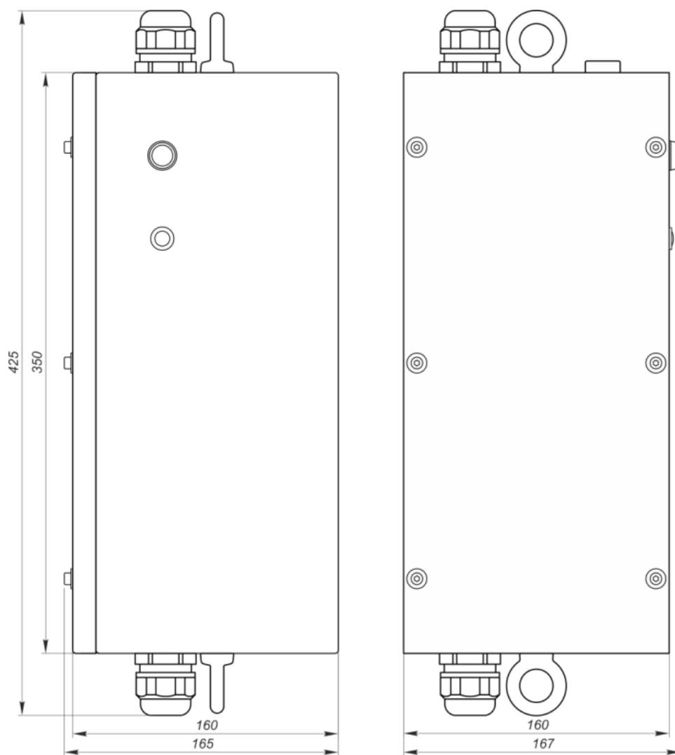
Рис. 7 Габаритный и монтажный чертеж.
