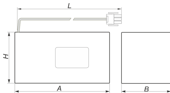
Рис. 5 Батарея BS-2P4S-IFpR-H-32/70-6,0/2F-HB300-MATE/N/LOK/3N-1 а27901
