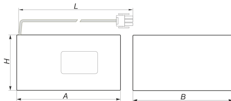
Рис.6 Батарея BS-4P4S-IFpR-H-32/70-6,0/4F-HB300-MATE/N/LOK/3N-1 а27899
