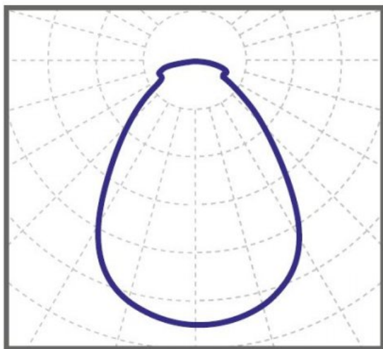
косинусная KCC 80°
