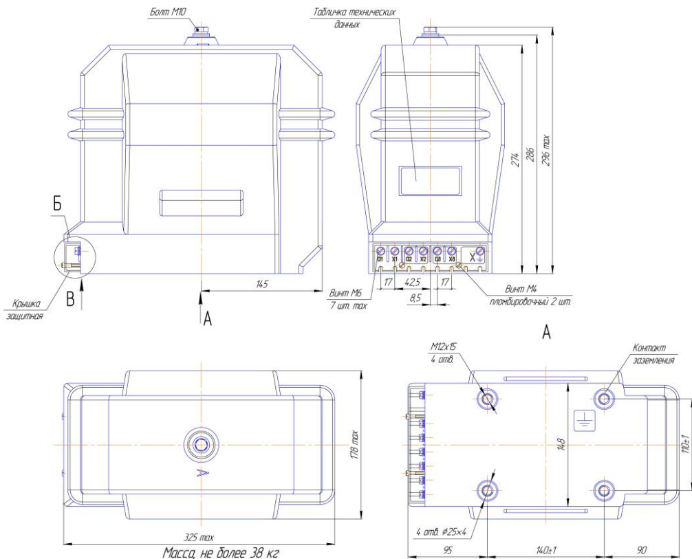
Рисунок А.4 – Габаритные, установочные, присоединительные размеры и масса трансформаторов ЗНОЛ-НТЗ-6(10)-02
