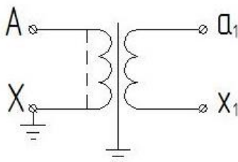
Рисунок Б.1 – Схема электрическая принципиальная трансформаторов с одной вторичной обмоткой без предохранителя
