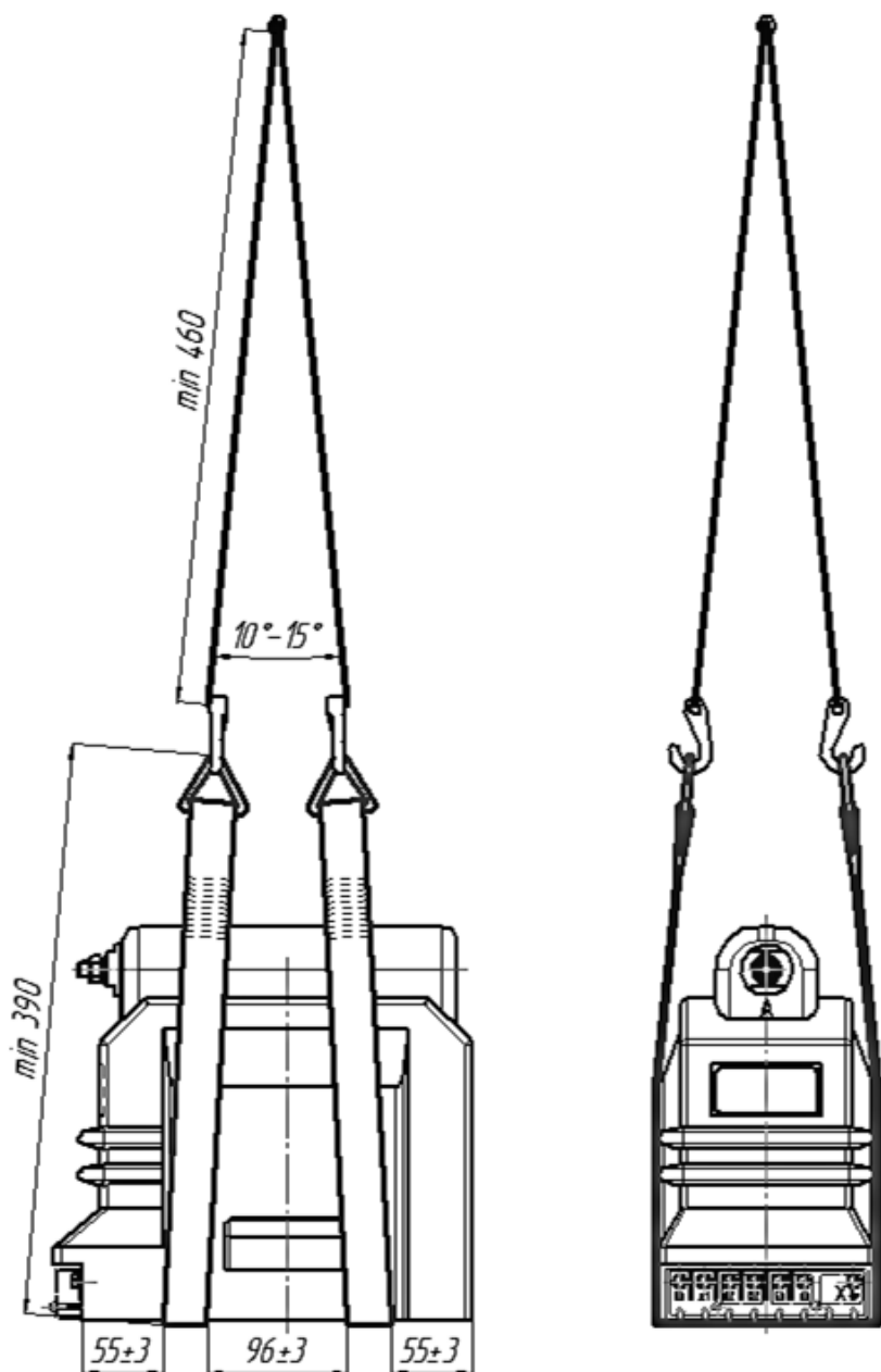
Рисунок В.1 – Схема строповки трансформаторов ЗНОЛ(П)-НТЗ-6(10) (-01, -02, -03, -05)
