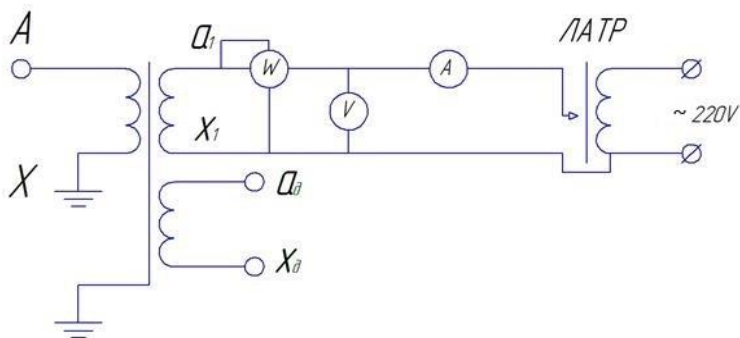
Рисунок 2 – Схема проведения испытания для трансформаторов с двумя вторичными обмотками: с одной основной и одной дополнительной
