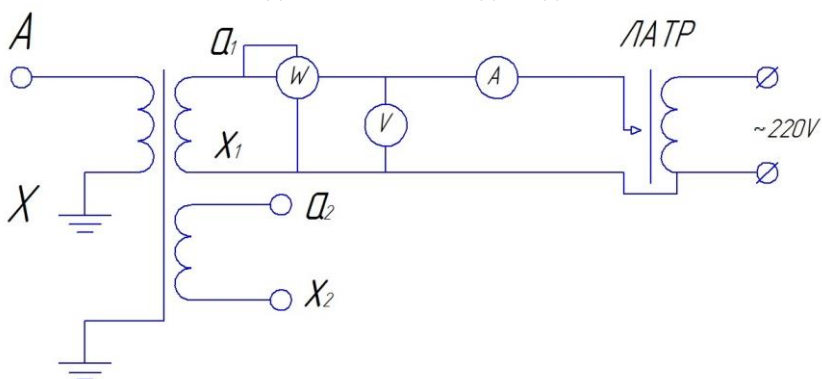
Рисунок 3 – Схема проведения испытания для трансформаторов с двумя основными вторичными обмотками
