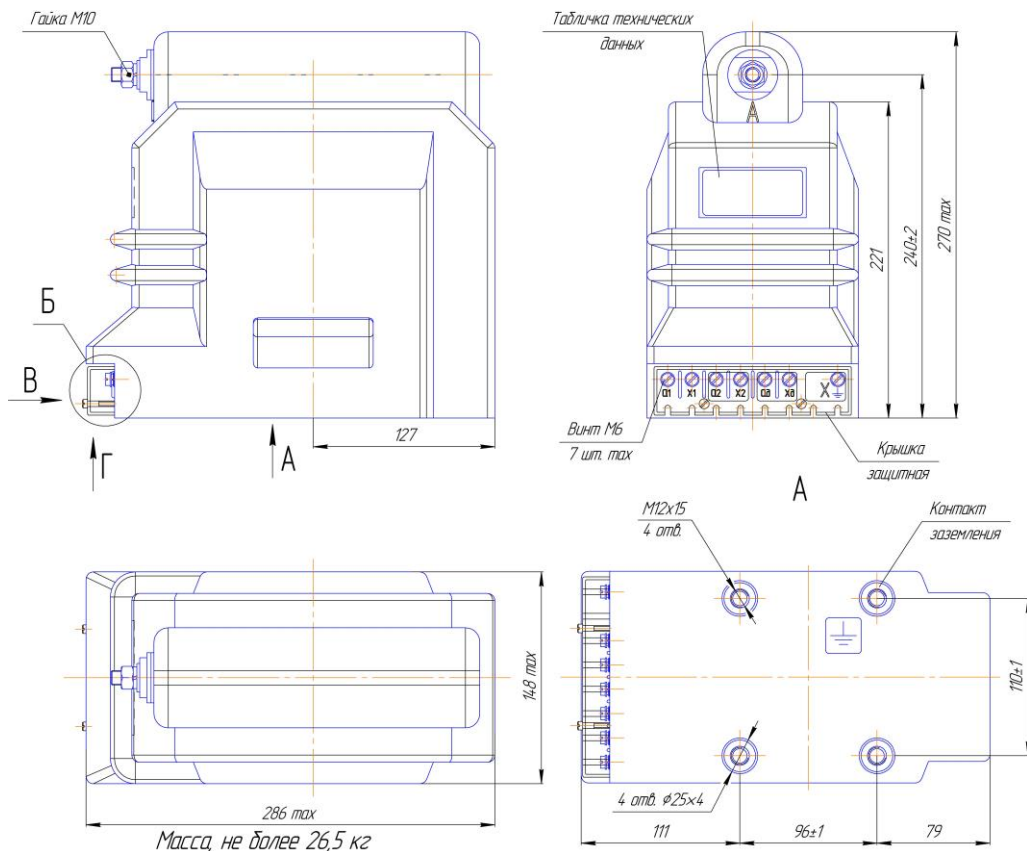
Рисунок А.2 – Габаритные, установочные, присоединительные размеры масса трансформаторов ЗНОЛП-НТЗ-6(10) и ЗНОЛП-НТЗ-6(10)-05
