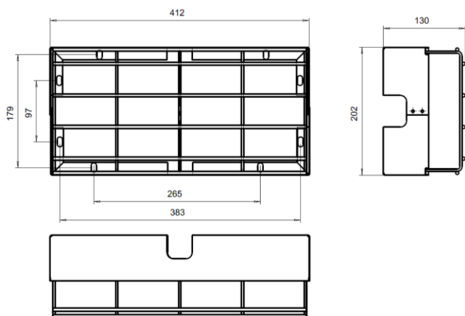
Рис. №4 Решётка защитная BS-R-1 (а2333)
